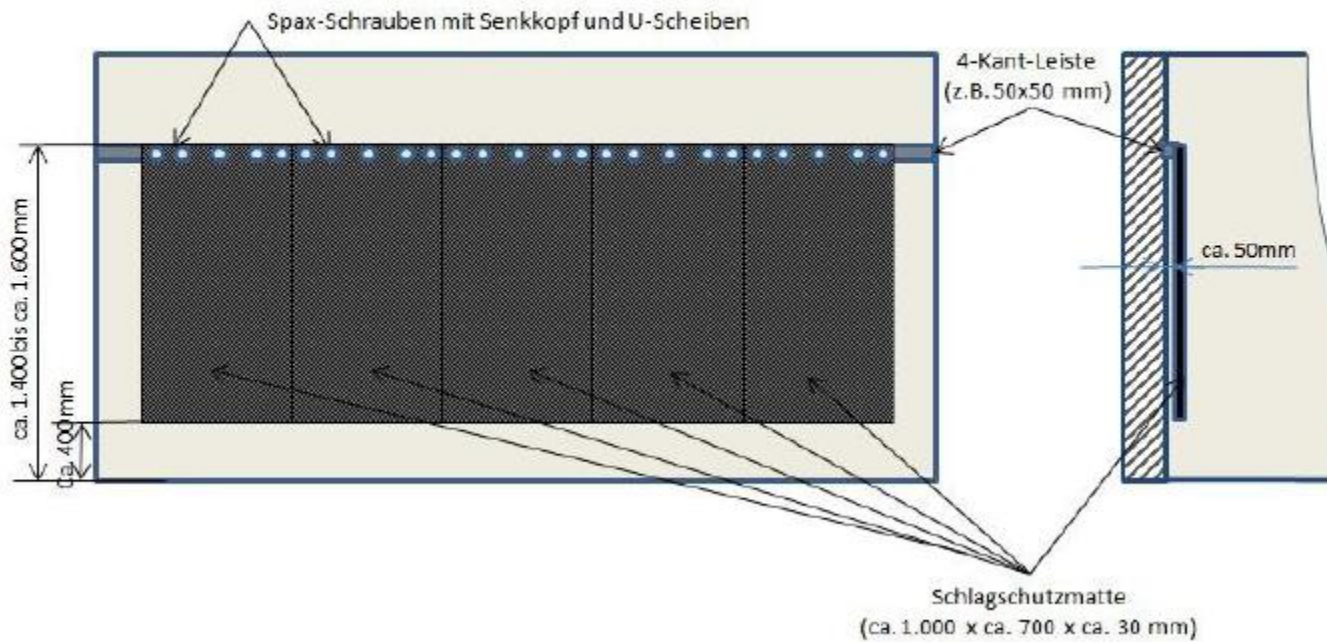
Seitenansicht: (Querschnitt)
